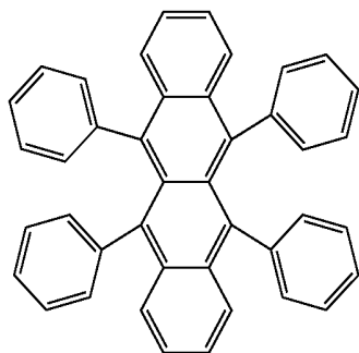
Rubrene
