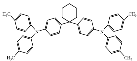
TPAC
