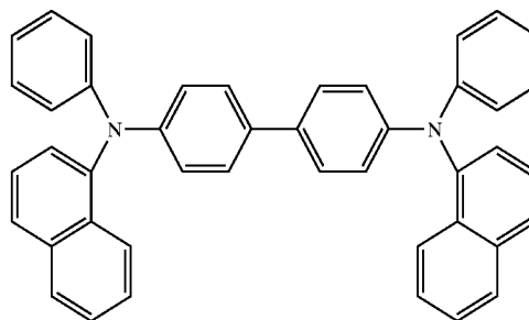
a-NPD
