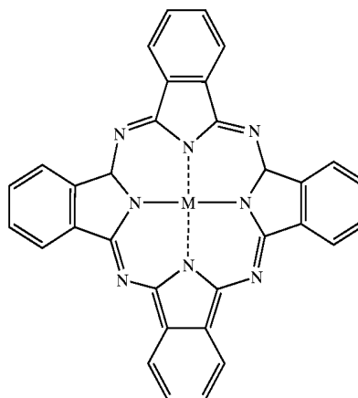
Pc-M
