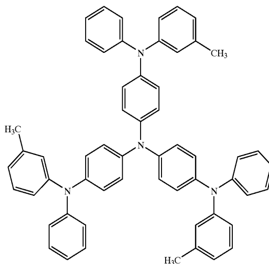
m-MTDATA
